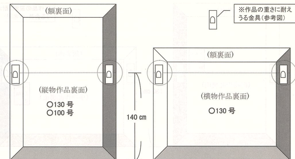
〔金具参考図〕
